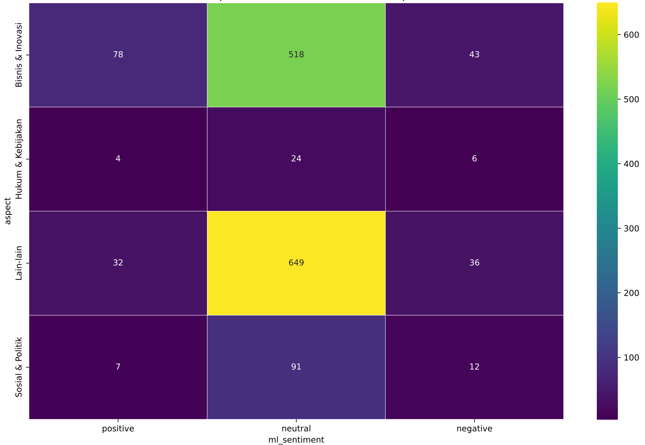
Heatmap Sentimen Berdasarkan Aspek
